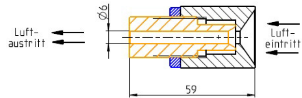
SCHNITT A-A
